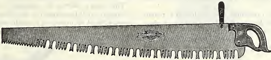
No. 222. Lance Tooth. 3 1/2—4—4 1/2 feet.
