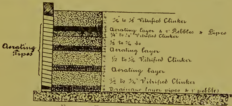
FIG. 24.—FILTERING MATERIAL.
