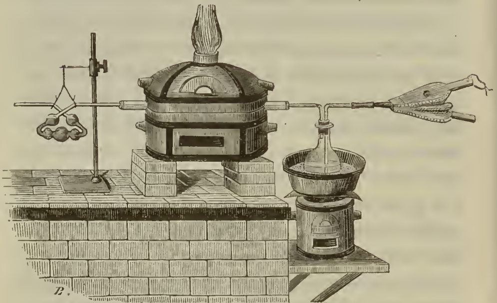
FIG. 2. — Appareil pour la recherche du chloroforme (1).
