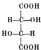
d-Weinsäure,
