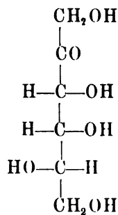
l-Tagatose.
