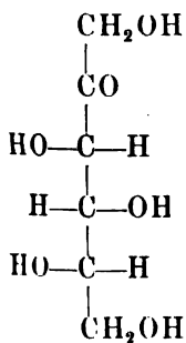
d-Sorbinose
