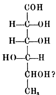
Rhamnose
