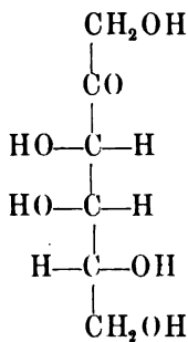
d-Tagatose
