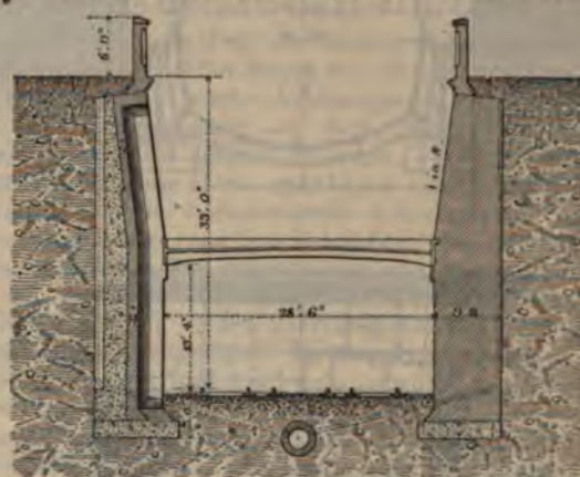
Fig. 15. Futtermauer mit gusseiserner Stützenabsteifung.
