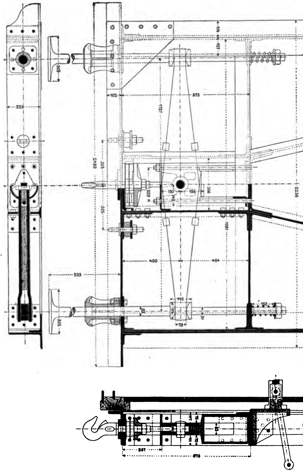
Fig. 75. Buffer- und Kupplungsvorrichtung der vierachsigen Metropolitan-Wagen.
