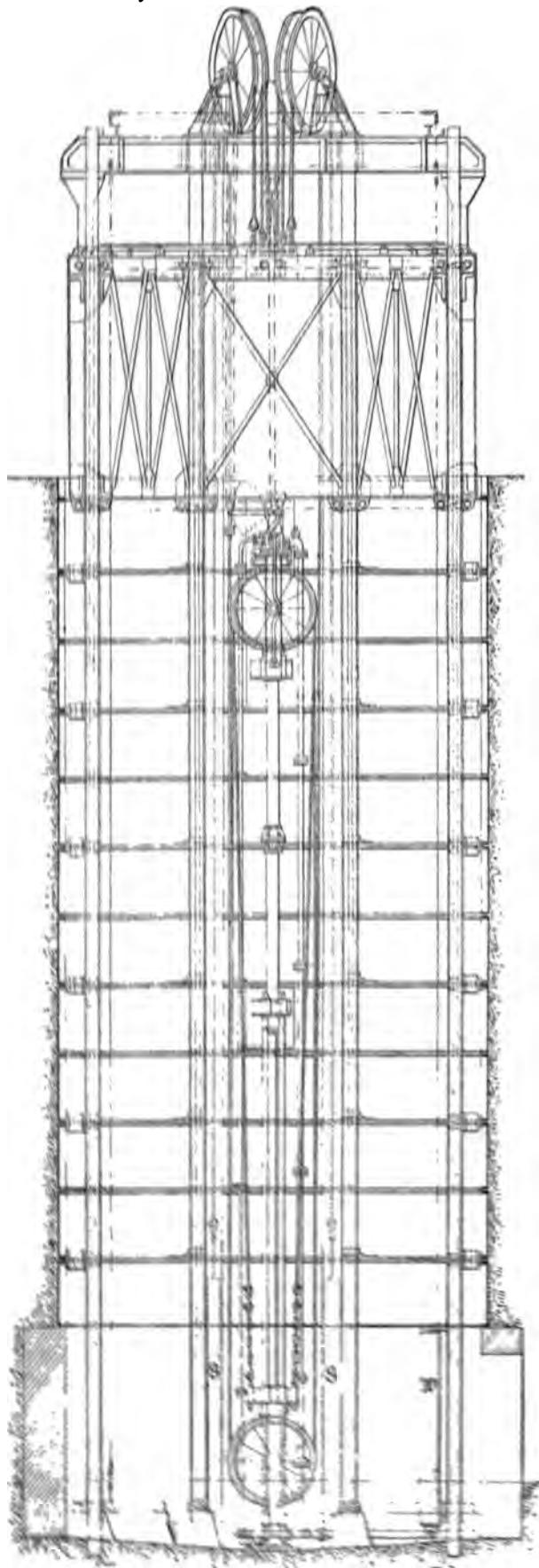
Fig. 129. Hydraulische Aufzüge.
