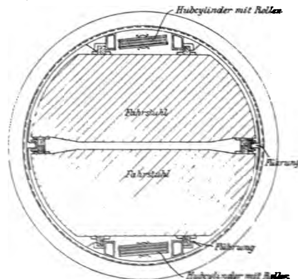
Fig. 130. Grundrissanordnung der hydraulischen Aufzüge.
