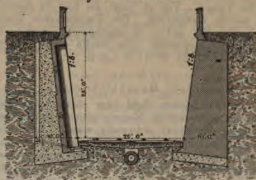
Fig. 14. Futtermauer.
