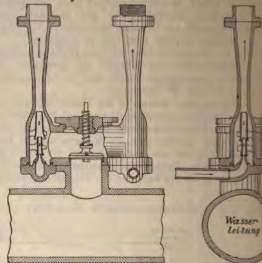
Fig. 137. Greathead-Ejektor.
