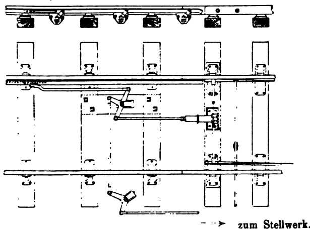
Fig. 44. Weichenverriegelung.
