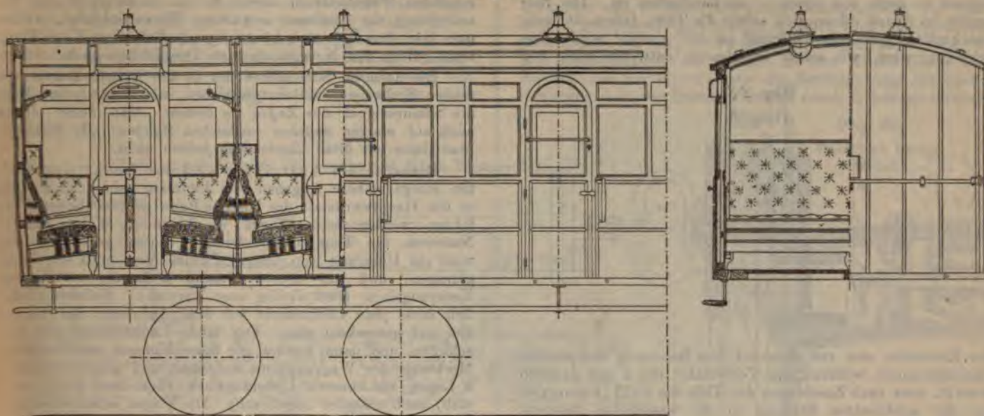
Fig. 94 und 95. Wagen I. Kl. (achträdrig) der Metropolitan-Bahn.
