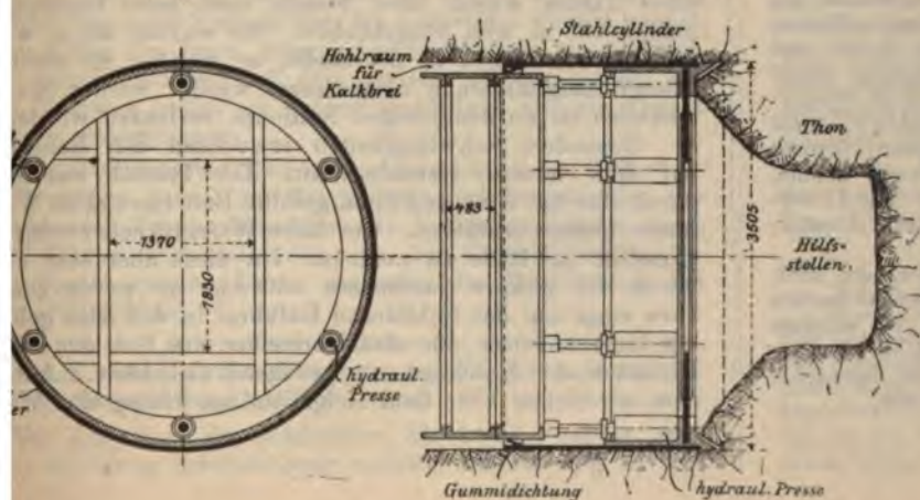
Fig. 123. Stahlschild zum Vortreiben des Tunnels.
