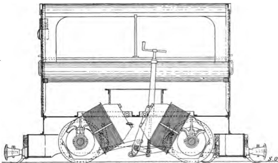
Fig. 155. Außere Ansicht der elektrischen Lokomotive.
