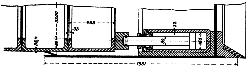
Fig. 125. Hydraulische Presse.
