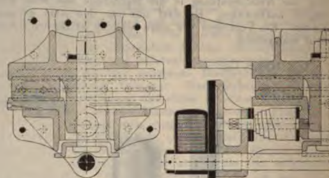
Lokomotiv-Drehgestell der Metropolitan-Bahn.
