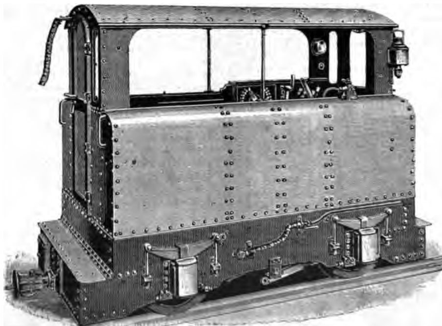
Fig. 155. Außere Ansicht der elektrischen Lokomotive.
