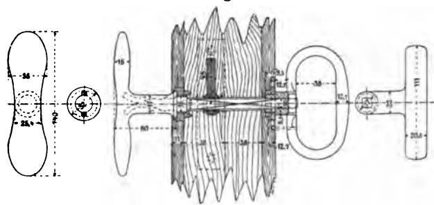
Fig. 96. Thürgriff.
