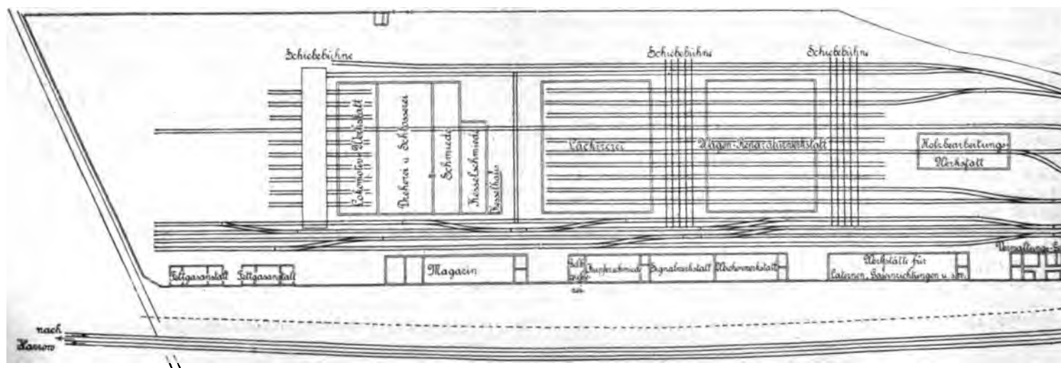
Grundriss der Neasdener Reparaturwerkstätte.
