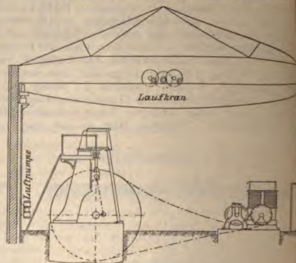
Fig. 141. Querschnitt des Maschinenhauses.
