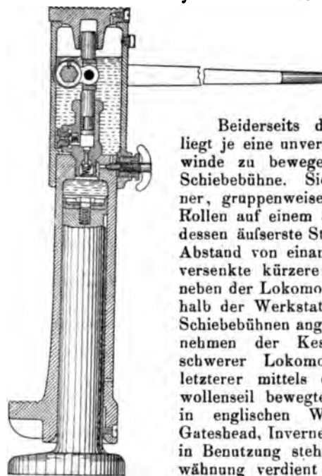
Fig. 107. Hydraulische Winde.
