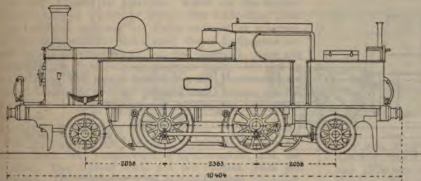
Untergrundlokomotive der London and North Western-Bahn.
