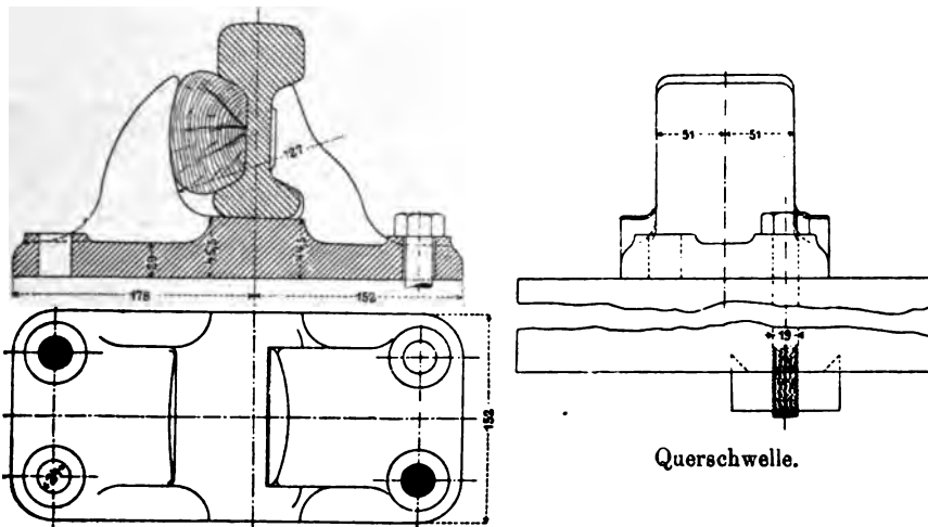
Fig. 40. Schiensstuhl.
