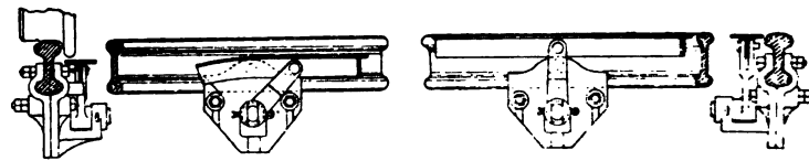
Fig. 46 a. Fig. 46 b. Weichen-Verschlusschiene.
