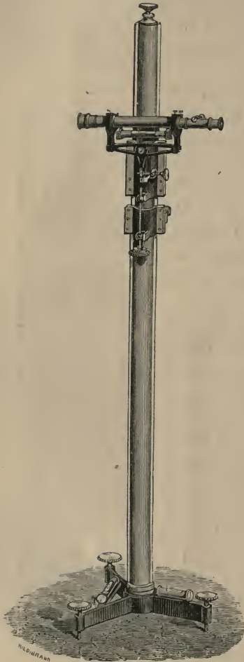
Fig. 111.—Cathetometer.
