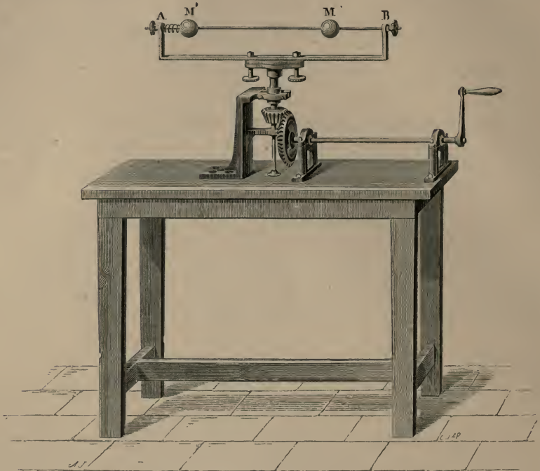
Fig. 37.—Centrifugal-force Apparatus.
