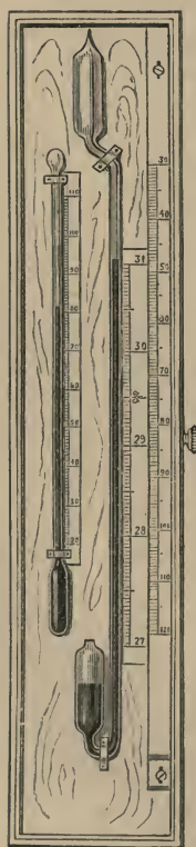
Fig. 117 Sympiesometer.
