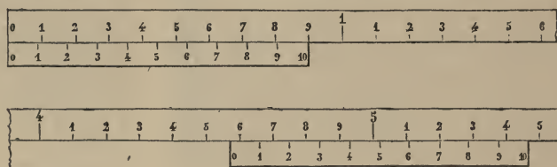
Fig. 114.—Vernier.
