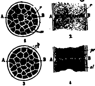
Figs. 34 á 37.—Desarrollo de una criba ( Cucurbita maxima ).—1, sección transversa: r , red celulósica; m , mallas rellenas de substancia albuminoidea.—2, sección longitudinal del vaso criboso atravesando la criba anterior por AB: r , fragmentos de la red seccionados.—3, sección transversa de una criba de más avanzada edad que la 1: p , perforaciones.—4, sección longitudinal de la anterior siguiendo la dirección AB: pr , protoplasma parietal; al , substancia albuminoidea atravesando las perforaciones.
