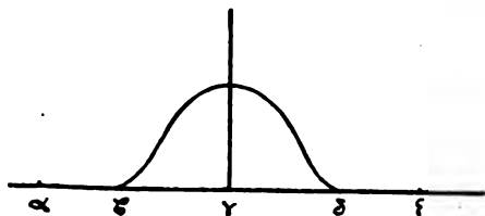
Fig. 193.—Curva explicativa de los fenómenos vitales en función de la temperatura.— \alpha , \beta , \gamma , \delta , \epsilon , temperaturas críticas; \gamma , óptimum de temperatura.
