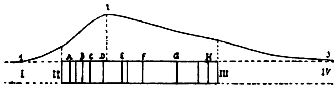
Fig. 89.—Curva de acción verdosa según las diversas radiaciones.—I-II, infra-rojo; II-III, espectro luminoso; III-IV, ultra-violado; A H, rayas principales del espectro; 1 y 3, acción clorofílica nula; 2, máximum de verdor cerca de la raya D.
