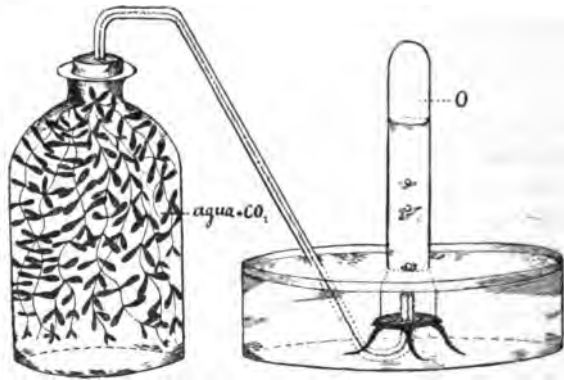
Fig. 202. — Planta de Callitriche stagnalis colocada en el interior de un recipiente con agua cargada de CO_2 . El recipiente se expone á la luz, con cuya influencia la planta citada desprende burbujas de oxígeno que se dirigen por el tubo vector ó de desprendimiento á la probeta.
