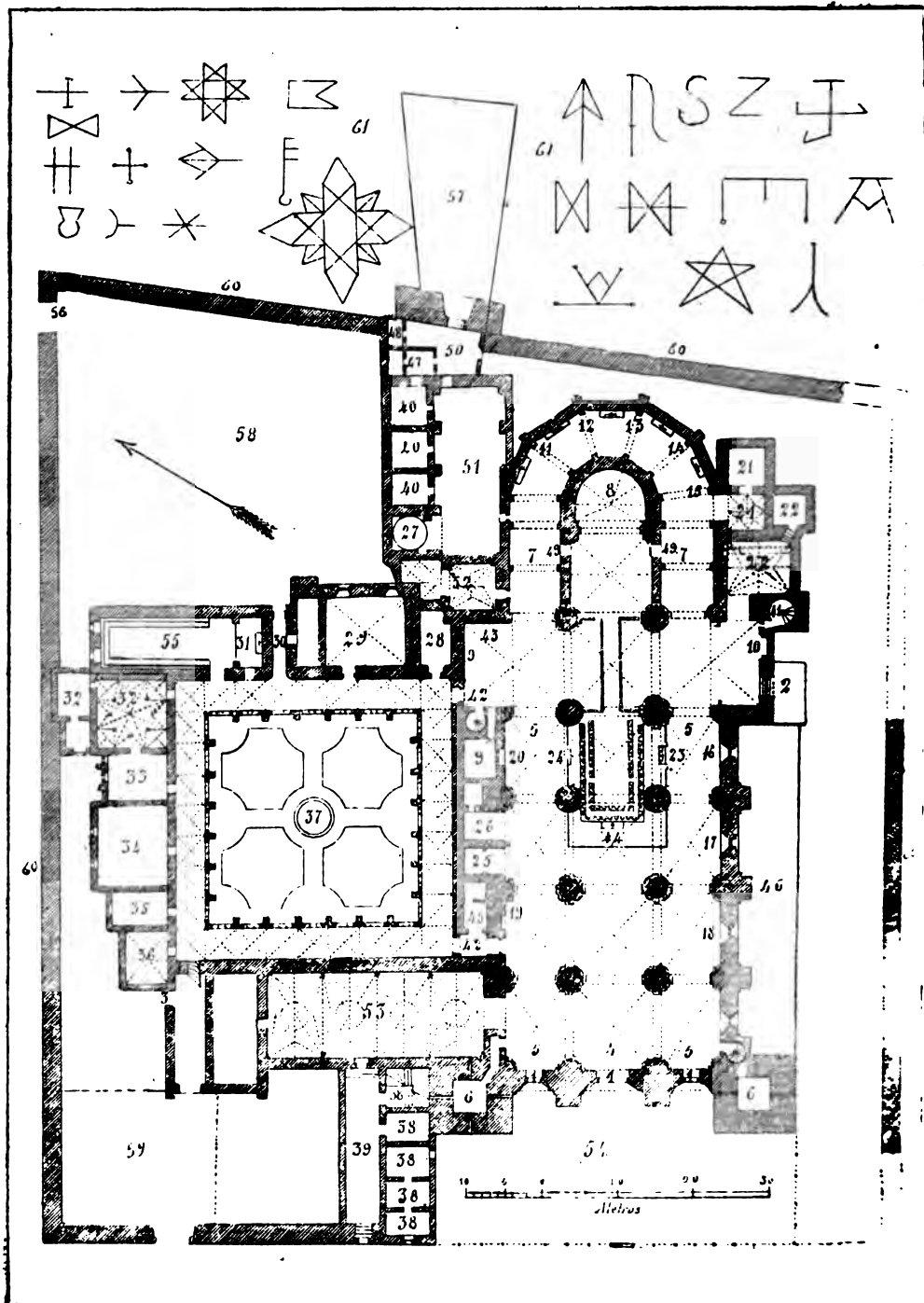
PLANO DE LA CATEDRAL DE SIGÜENZA
