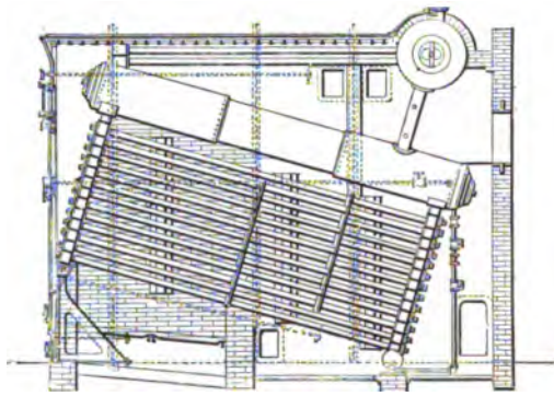
ZELL . . . . . 3750 H.-P.
